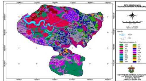
Gambar 4. Peta Sebaran Koefisien Limpasan Permukaan
