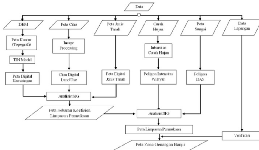
Gambar 3. Bagan Alir Metodologi studi.
